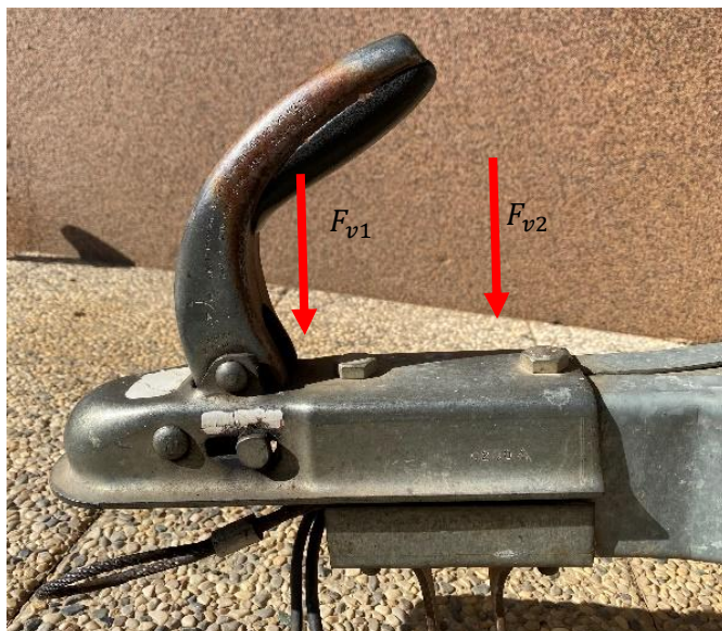
Slika 3: Sila na vijaka kljuke, Vir: Đukić 2025
