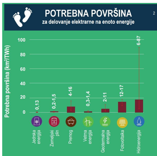
Slika 4: Poraba površine za postavitev elektrarne glede na oddano TWh elektrike (Vir: A. Trainor et al., 2016, stran 49)
