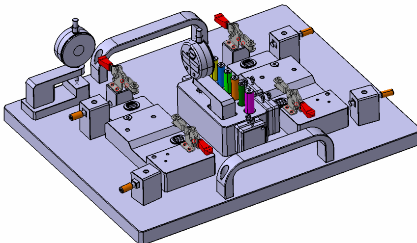
Slika 2: Atributivna kontrolna priprava CAD model
